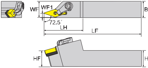
寸法 Dimension(mm)
