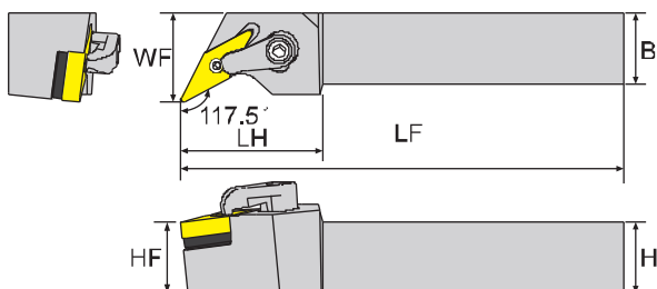
寸法 Dimension(mm)
