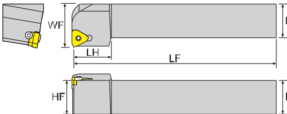
寸法 Dimension(mm)
