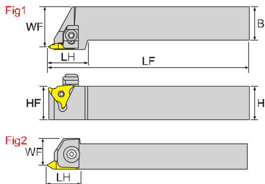
寸法 Dimension(mm)
