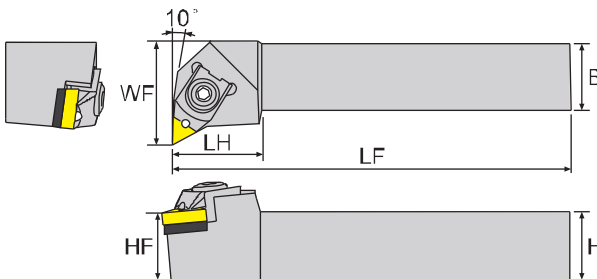
寸法 Dimension(mm)
