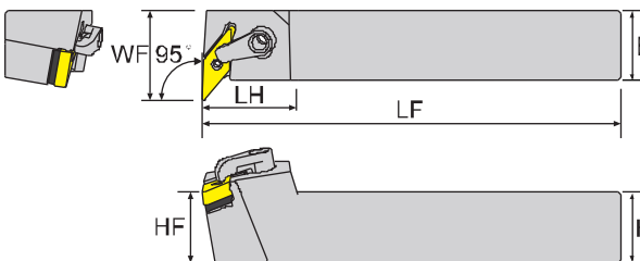
寸法 Dimension(mm)
