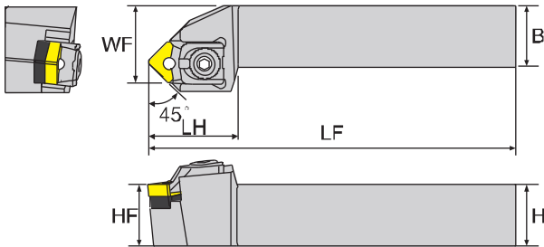
寸法 Dimension(mm)
