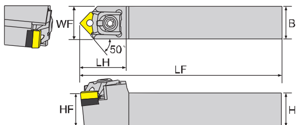
寸法 Dimension(mm)
