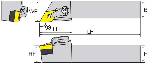
寸法 Dimension(mm)
