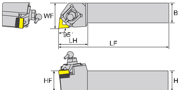
寸法 Dimension(mm)
